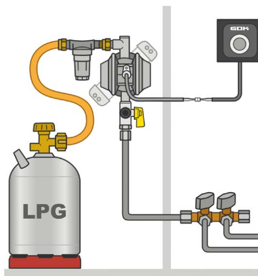
Caramatic BasicOne avec dispositif d'essai
